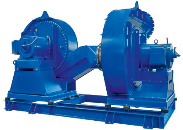
Gasdichter Radialventilator in zweistufiger Ausführung für den Transport von Wasserstoff.
